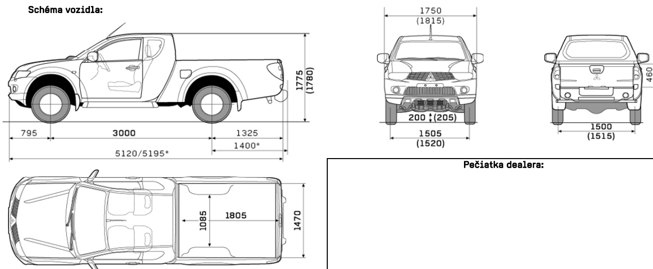
Schéma vozidla:
