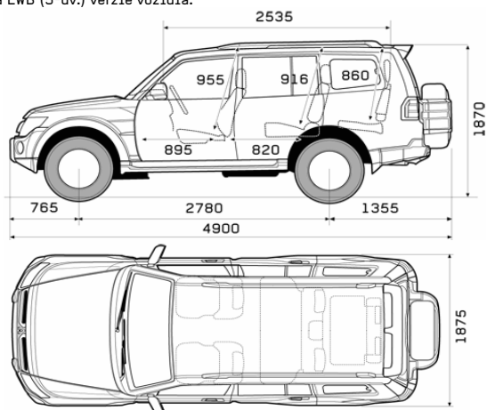
Schéma LWB (5-dv.) verzie vozidla:
